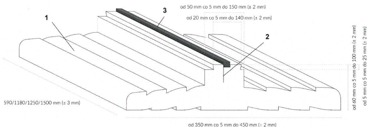
Rys. B1. Profil okienny ECOSILL – pełny
